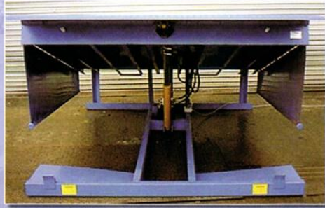
وحدة تعديل المنسوب ( Dock Leveler )
